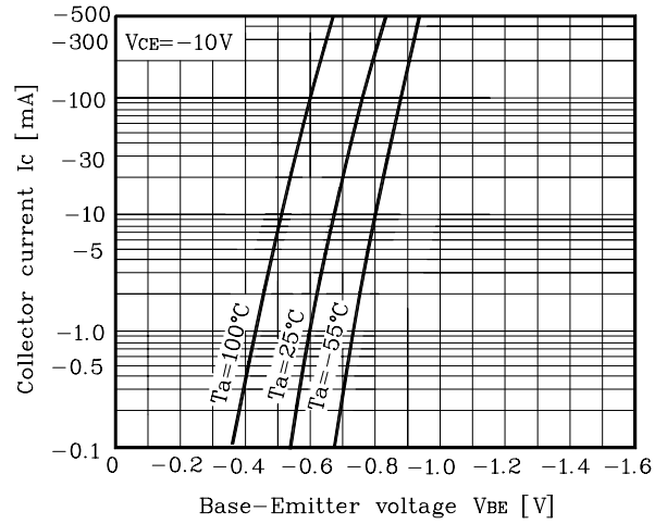
Fig. 2 I_C - V_{BE}
