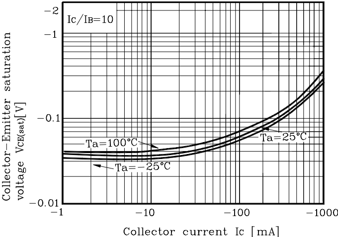
Fig. 5 V_{CE(sat)} - I_C
