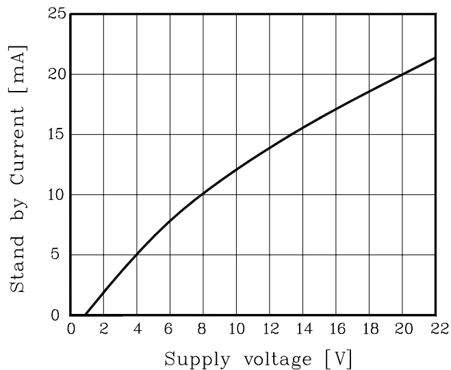
Fig. 1 V_{CC} - I_{SB}
