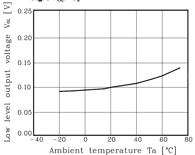
Fig. 6 V_{OL} - T_a
