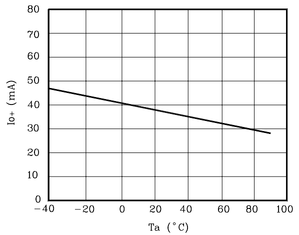
Fig. 4 I_O-T_a
