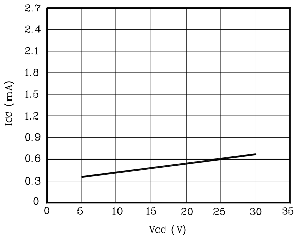
Fig. 1 I_{CC}-V_{CC}
