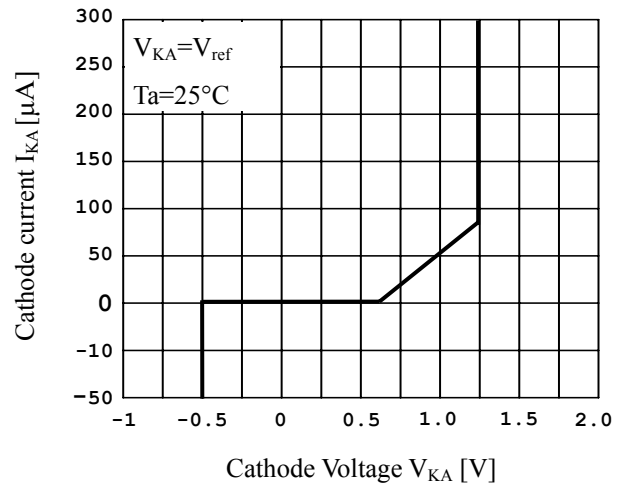
Fig.5 I_K vs V_{KA} (2)
