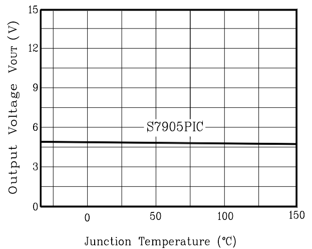
Fig. 4 V_{OUT} - T_j
