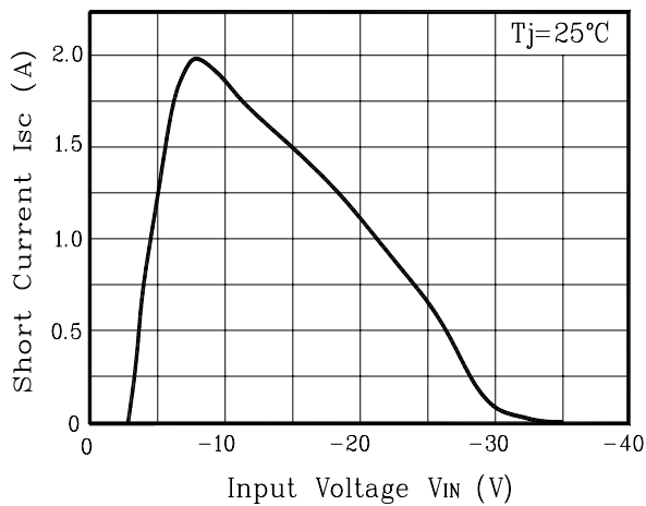
Fig. 5 I_{SC} - V_{IN}
