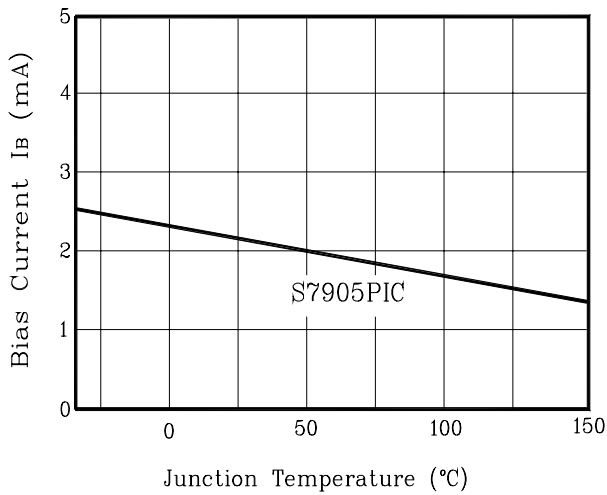
Fig. 3 I_B - T_j
