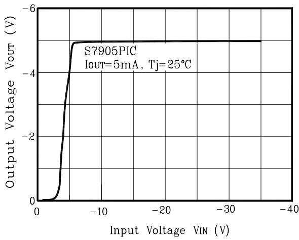
Fig. 1 V_{OUT} - V_{IN}
