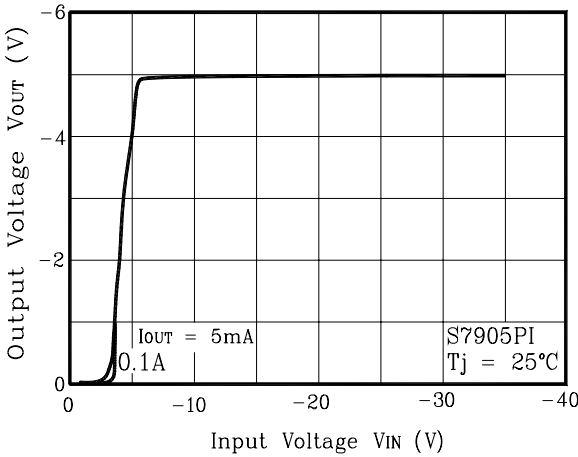
Fig. 1 V_{OUT} - V_{IN}
