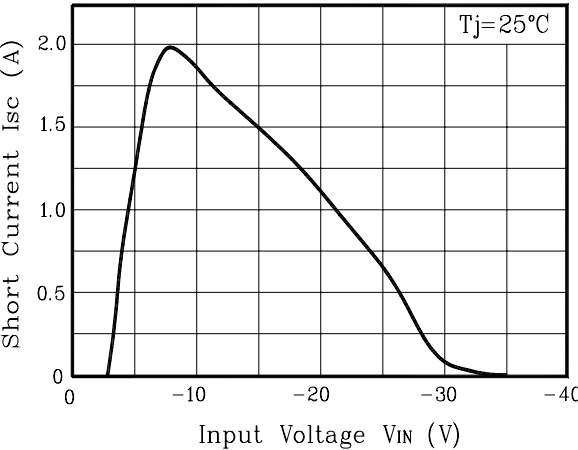
Fig. 5 I_{SC} - V_{IN}
