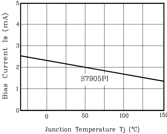
Fig. 3 I_B - T_j
