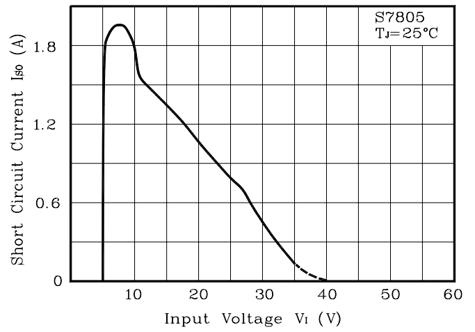
Fig. 8 I SO vs. V i
