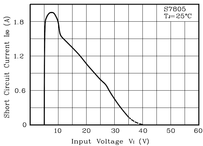
Fig. 8 I SO vs. V i
