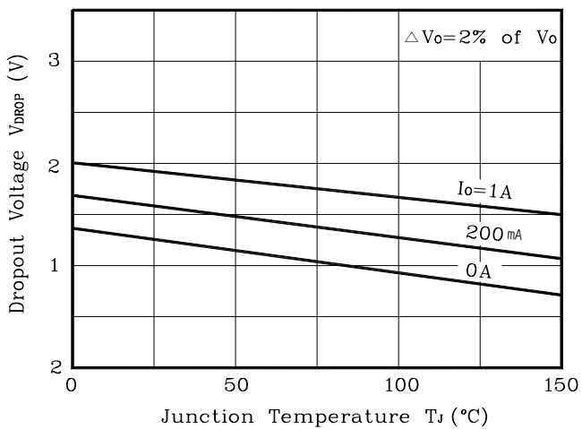
Fig. 5 V_{DROP} vs. T_J
