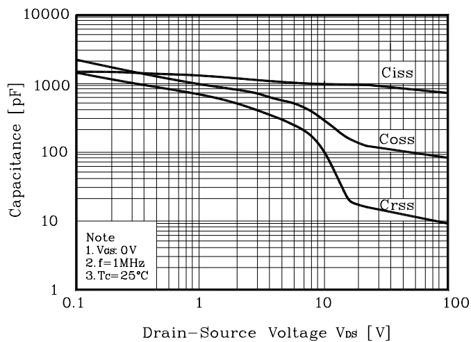
Fig. 5 Capacitance - V_{DS}
