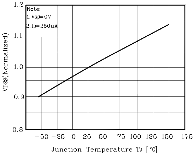
Fig. 7 V_{DSS} - T_J
