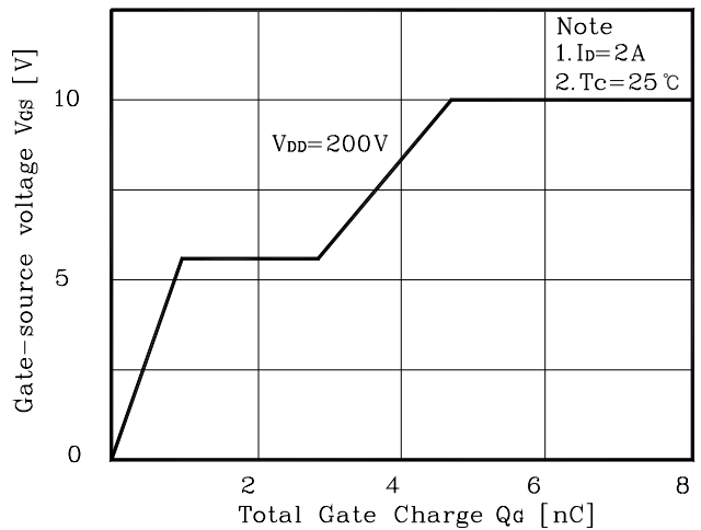
Fig. 6 V_{GS} - Q_G
