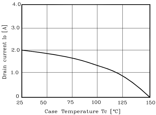
Fig. 9 I_D - T_C
