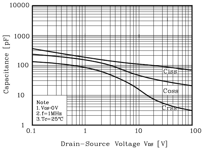
Fig. 5 Capacitance - V_{DS}
