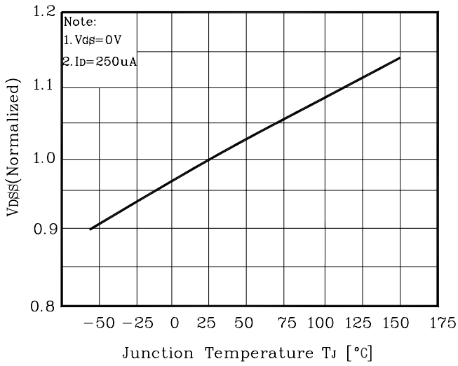
Fig. 7 V_{DSS} - T_J
