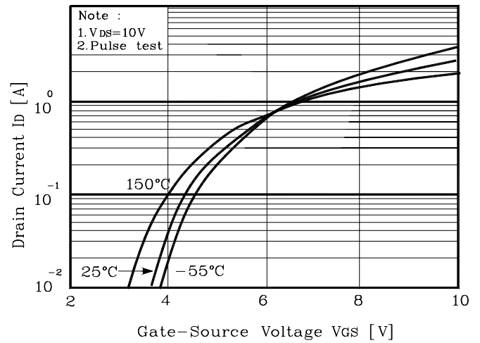
Fig. 2 I_D - V_{GS}
