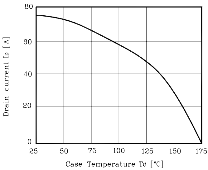
Fig. 9 I_D - T_C
