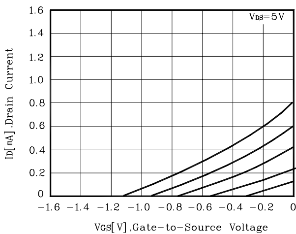
Fig. 5 V_{GS(Off)} - I_{DSS}
