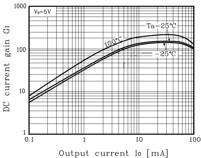
Fig. 3 G_1 - I_o
